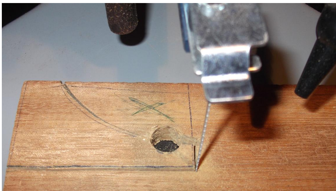
Κοπή τμήματος σε επιτραπέζια σέγα. Διάνοιξη οπής με τρυπάνι διαμέτρου 12 mm
