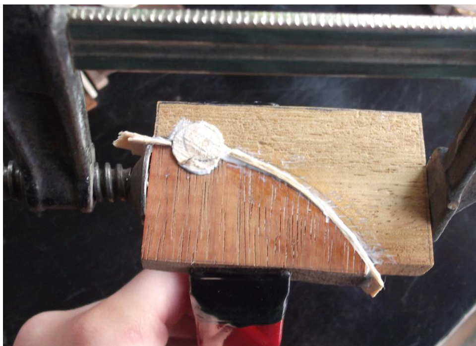
Συγκόλληση επιμέρους τμημάτων και συγκράτηση με σφιγκτήρες.
