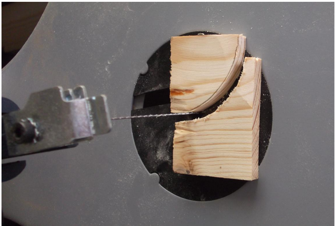
Κοπή των καμπύλων τμημάτων σε επιτραπέζια σέγα
