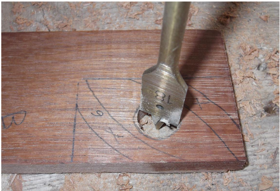
Διάνοιξη κεντρικής οπής με φτερό No 18
