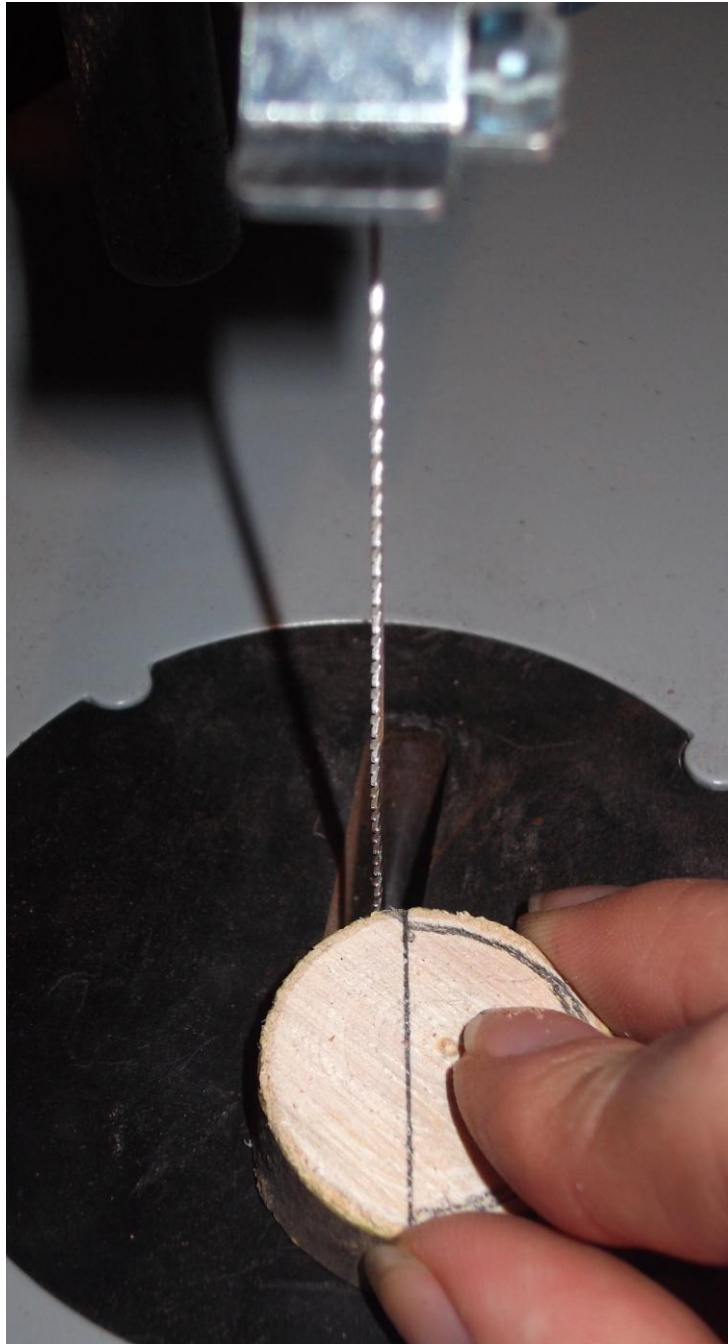
Κοπή σοκορου σε επιτραπέζια σέγα
