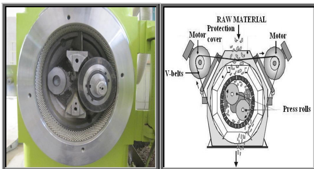
Εικόνα 5: Μηχανή pellet με μήτρα τύπου πυρήνα.
