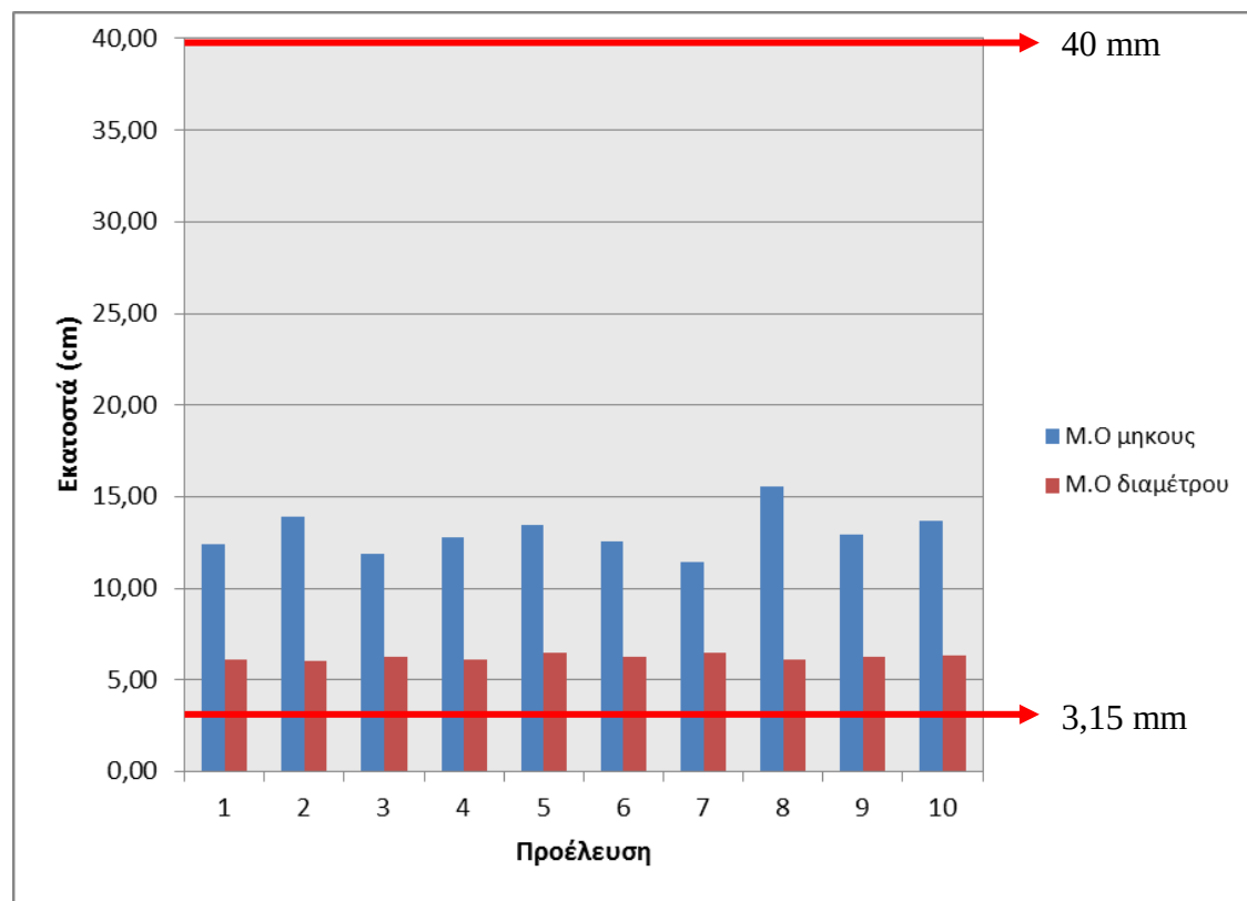
Εικόνα 27: Συγκεντρωτικό γράφημα μέσων όρων μήκους και διαμέτρων των δειγμάτων.
