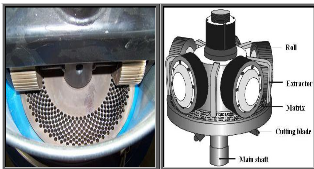
Εικόνα 4: Μηχανή pellet με επίπεδη μήτρα.
