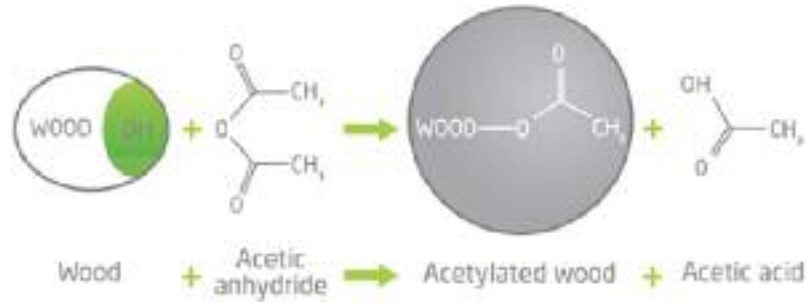
Σχήμα 1: Αντίδραση του ξύλου με οξικό ανυδρίτη
