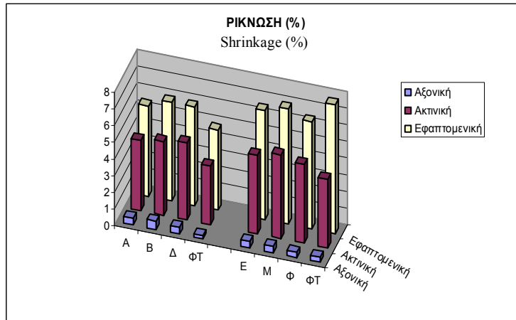
Σχήμα 4. Ρίκνωση δοκιμίων μετά την πυρκαγιά και τιμών που αναφέρονται στη βιβλιογραφία.
